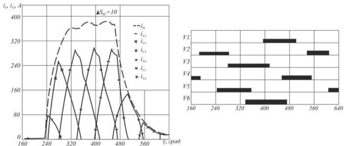
Рис. 3. Токи вентилях, нагрузки и циклограмма работы выпрямителя в режиме, близком к короткому замыканию
