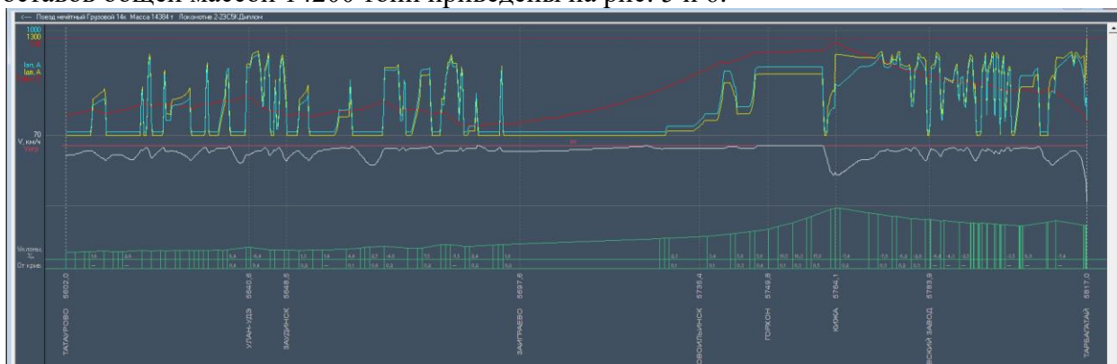
Рис. 5. Результаты тягового расчета состава массой 14200 тонн в нечетном направлении
