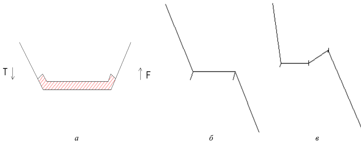
Рис. 2. Схемы участков в режиме торможения: a – вредной ямы; б – вредного уступа; в – горба у подножия вредного уступа Fig. 2. Schemes of sections in braking mode: a – harmful pit; b – harmful ledge; c – hump at the foot of harmful ledges
