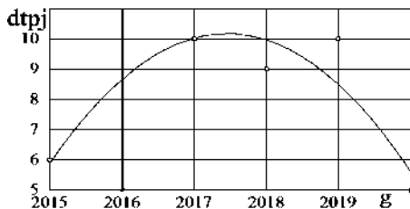
Рис. 7. Динамика численности дорожно-транспортных происшествий на железнодорожных переездах Иркутской области
