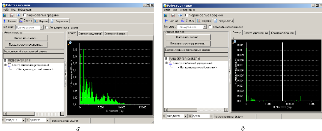
Рис. 10. Спектр огибающей:
