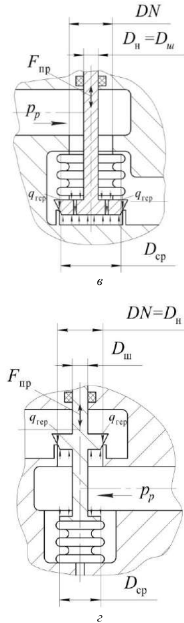
Рис. 3. Схемы разгруженного клапана: а, б – разгрузка поршневого типа; в, г – разгрузка сильфонного типа ( F_{\text{пр}} – усилие со стороны привода, D_{\text{н}} – диаметр неразгруженной части, D_{\text{р}} – диаметр разгруженной части, D_{\text{ш}} – диаметр штока Fig. 3. Schemes of the unloaded valve: a, b – piston type unloading; c, d – bellows type unloading ( F_{\text{пр}} – force from the drive side, D_{\text{н}} – diameter of the unloaded part, D_{\text{р}} – diameter of the unloaded part, D_{\text{ш}} – diameter of the stem)
