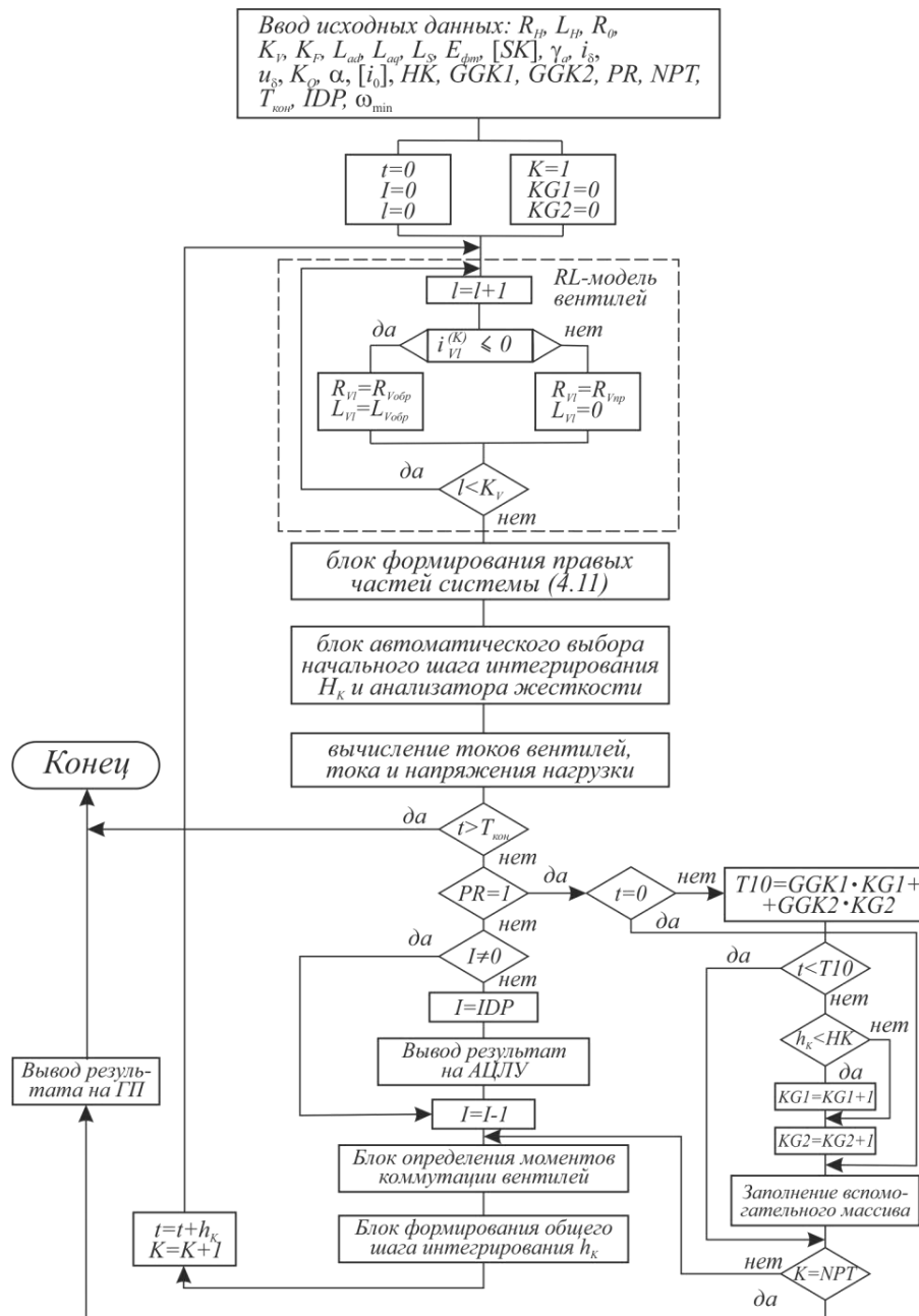
Рис. 2. Алгоритм цифровой модели вентильного магнетоэлектрического генератора
