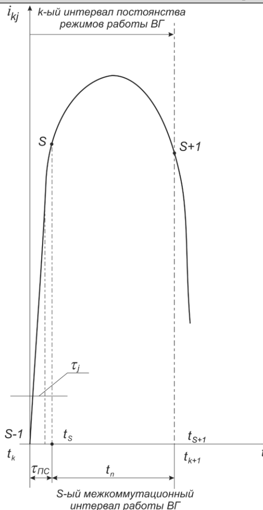
Рис. 1. Кривая тока через вентиль, поясняющая разнотемповость его производной Fig. 1. A current-through-valve curve illustrating the different-tempo character of its derivative
