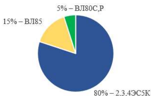
Рис. 4. Доля выявленных трещин в остовах тяговых электродвигателей НБ-514, приходящаяся на разные серии электровозов
