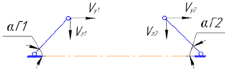
Рис. 3. Кинематическая схема относительных скоростей Fig. 3. Kinematic scheme of relative velocities
