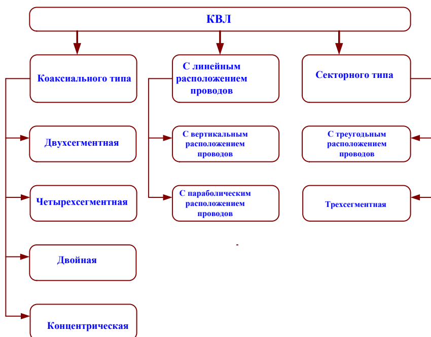
Рис. 4. Классификация компактных высоковольтных линий
